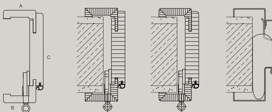
A : habillage décoratif
